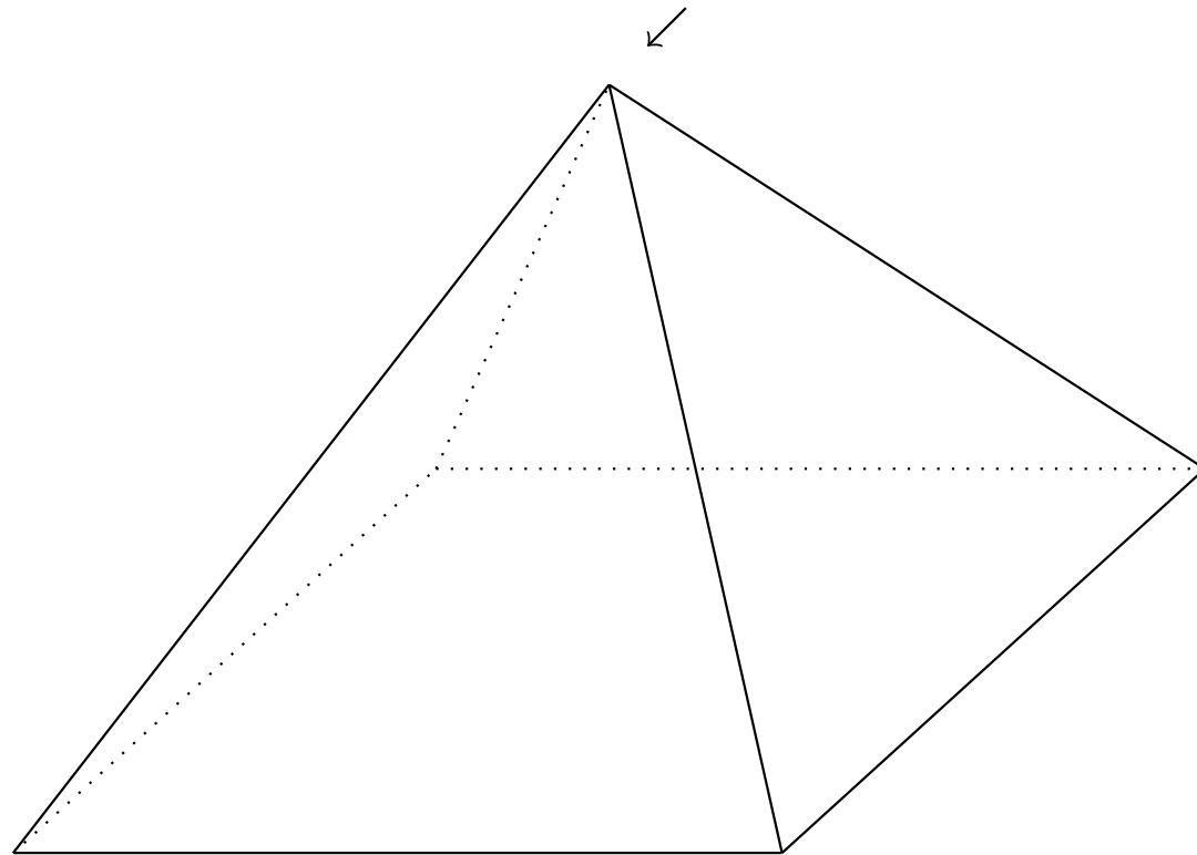
Figure: Eine degenerierte Lösung im \mathbb{R}^3 .
